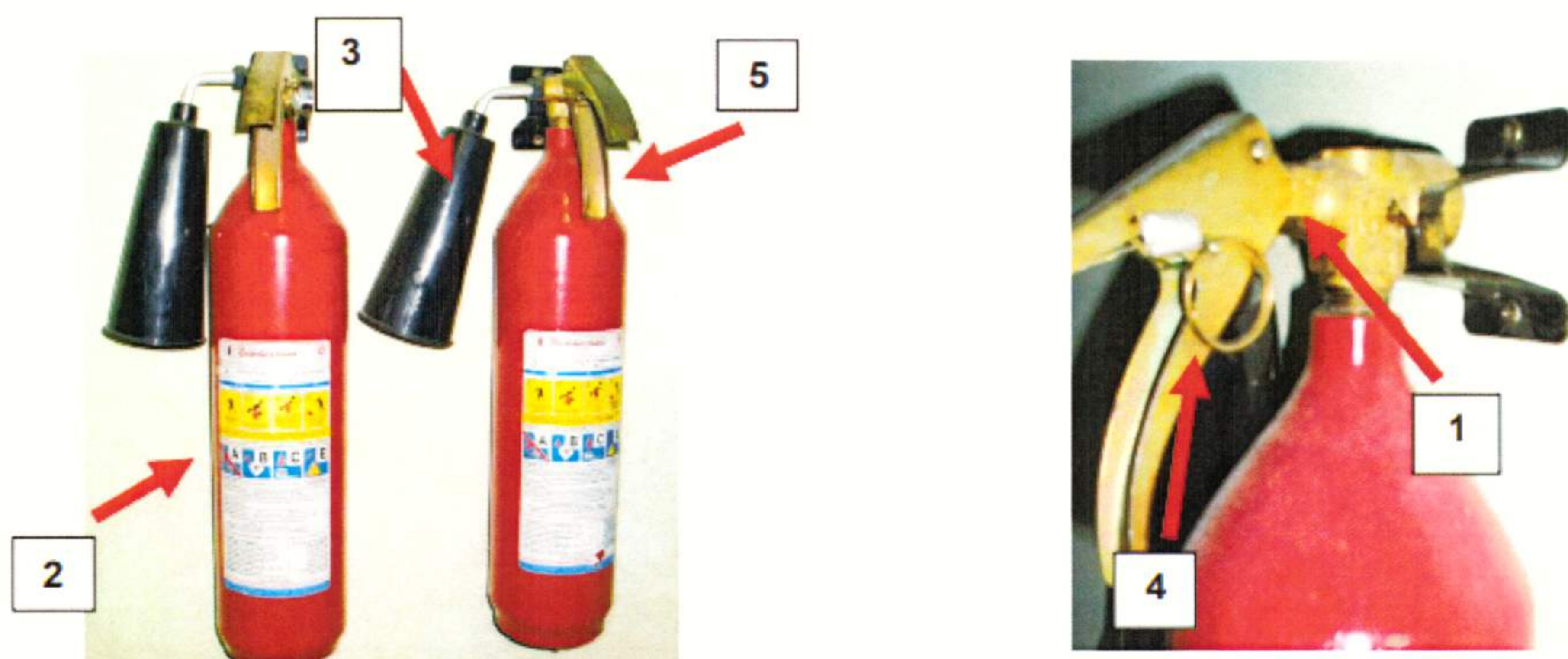
Рисунок 5 - Углекислотный огнетушитель типа ОУ-3
