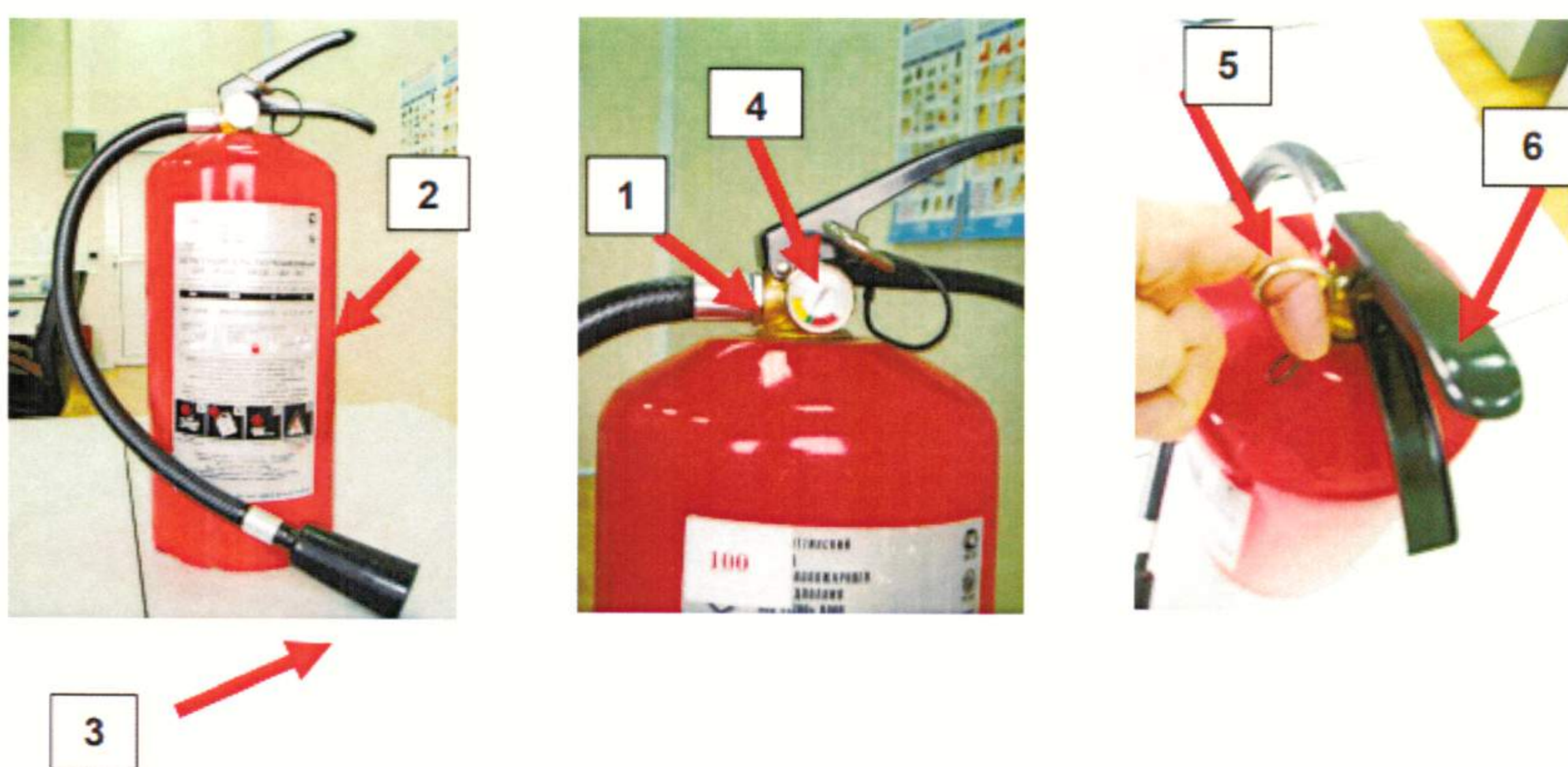
Рисунок 4 - Порошковый огнетушитель типа ОП-4(з)
