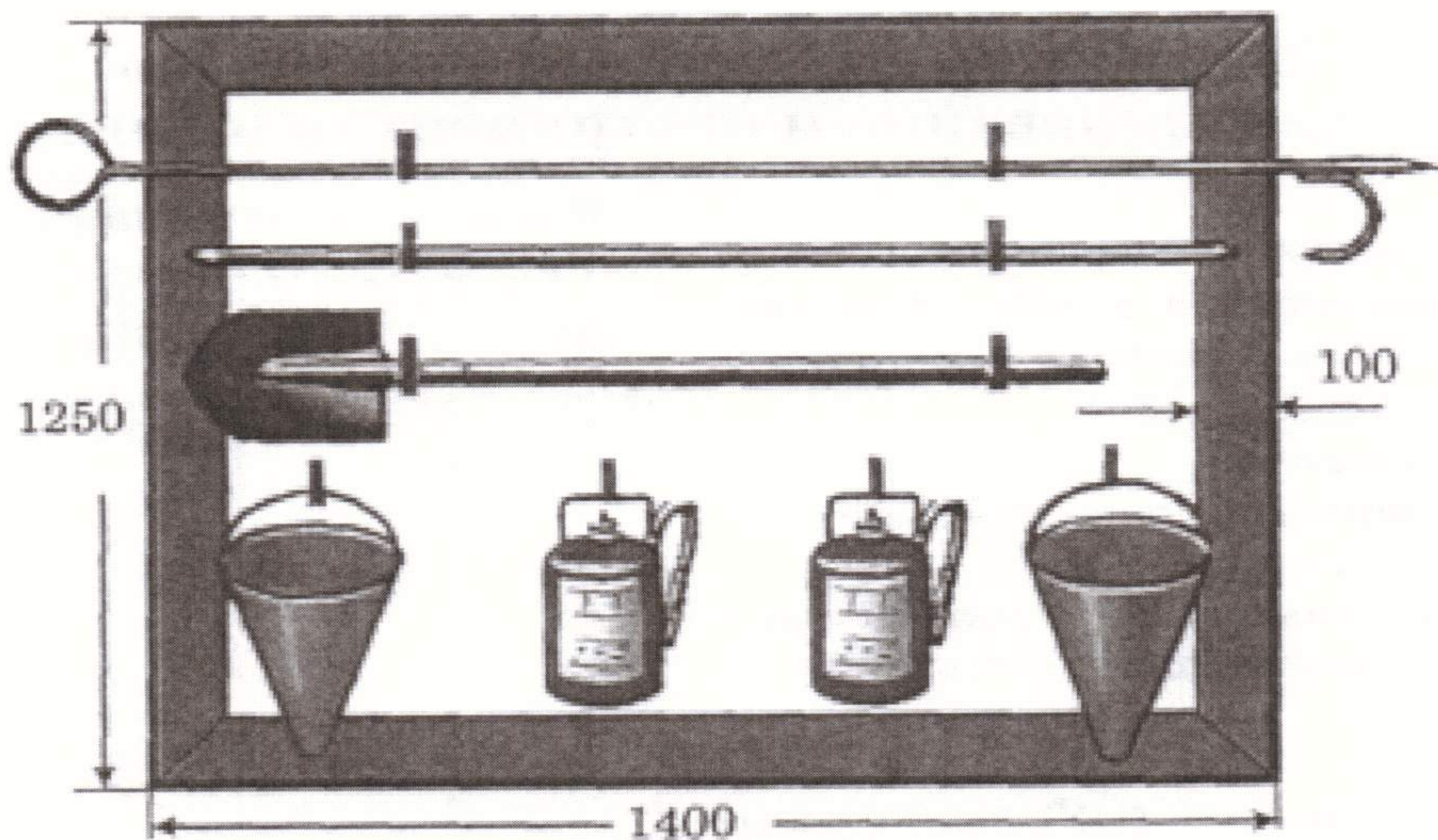
Рисунок 6 - Пожарный щит открытого типа
