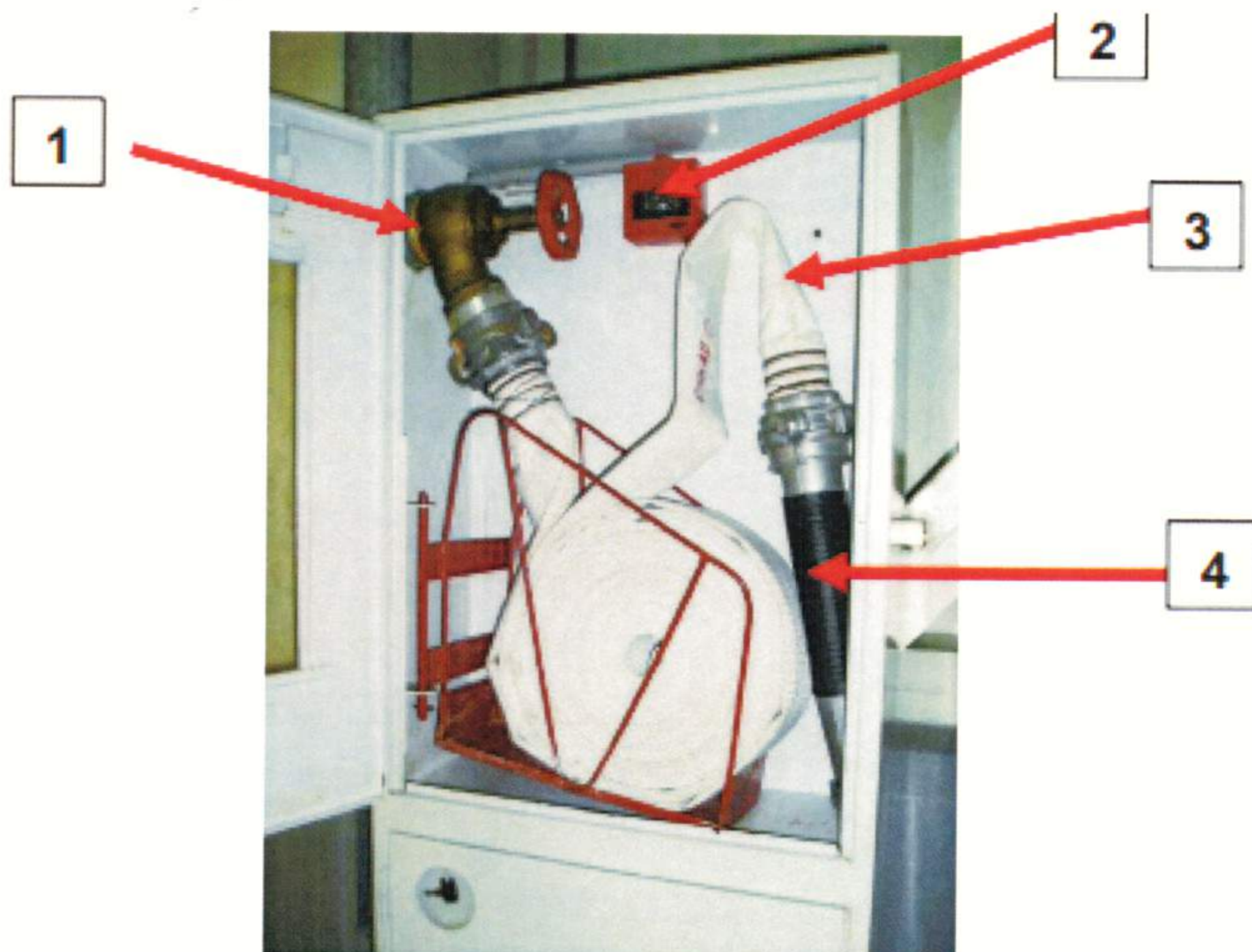
Рисунок 7 Внутренний пожарный кран
