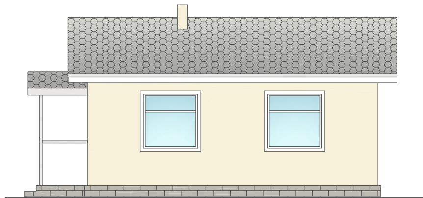
Фасад в осях А-Б.
