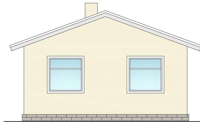
Фасад в осях 2-1.
