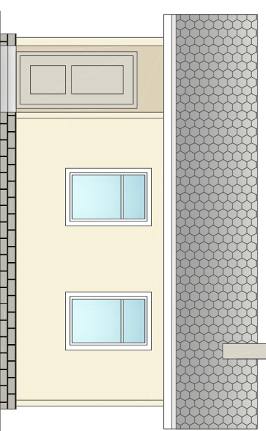
Фасад в осях А-В.
